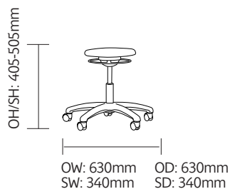
MSGL02 - Round Stool PU Seat
